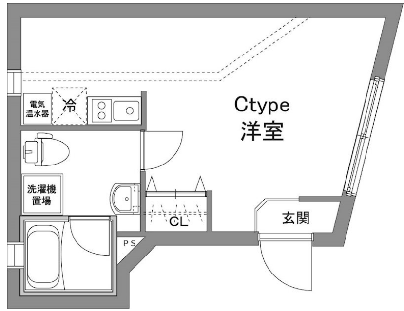
【間取り図】
